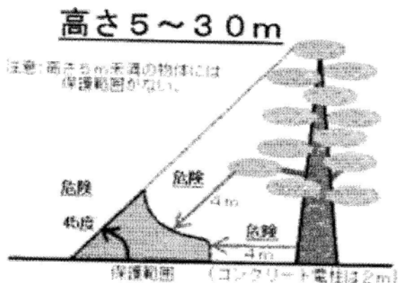
図 4 樹木周辺の落雷保護範囲
